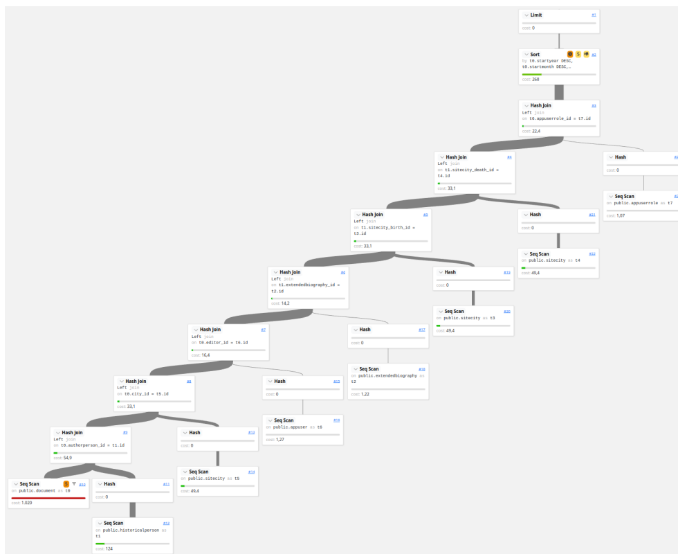
Abbildung 5.1: Visualisierung EXPLAIN
